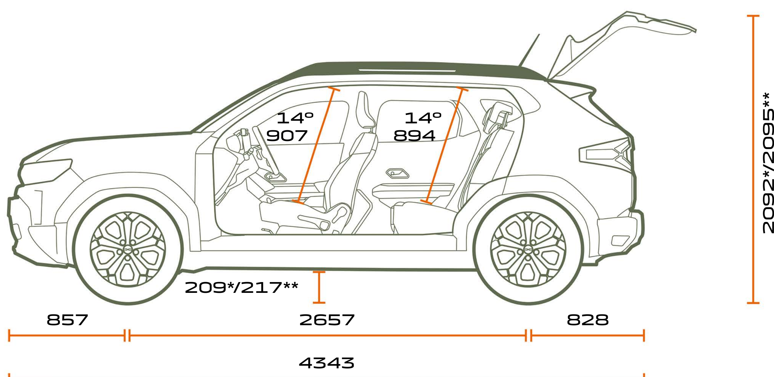
VAADE KÜLJELT
