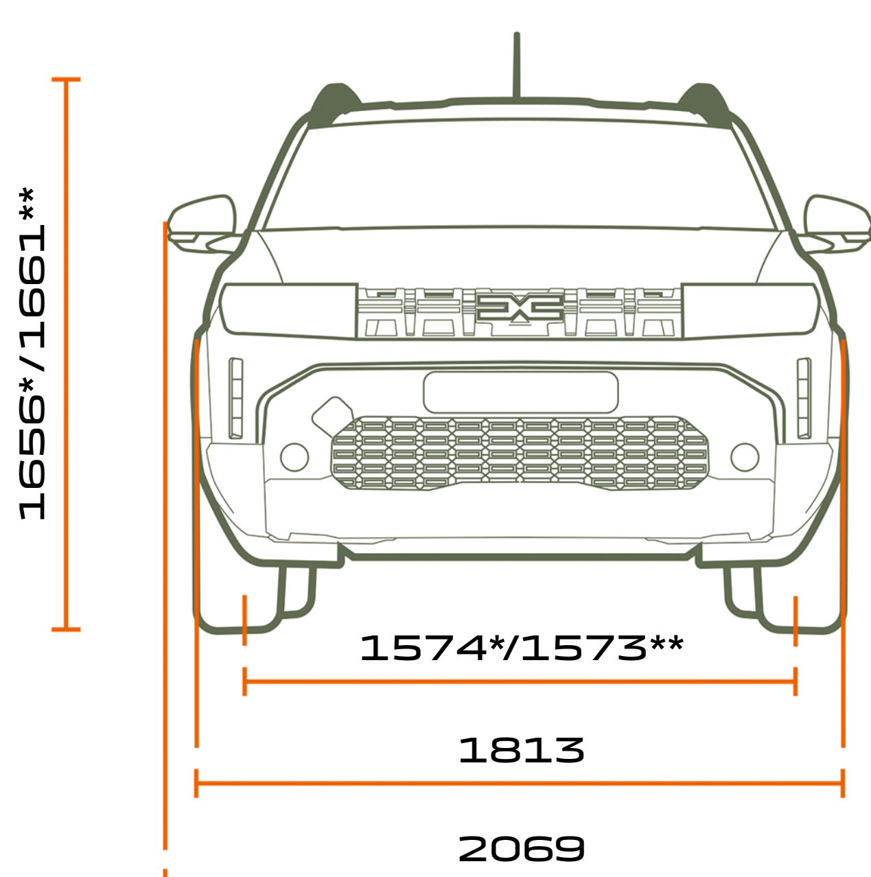
VAADE EEST
